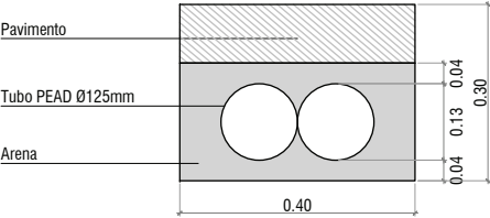
CANALIZACION DE 2 BAJO ACERA 1/10 (cotas en metros)
