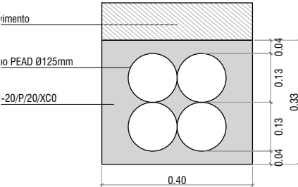
CANALIZACION DE 2 BAJO ACERA 0 (cotas en metros)
