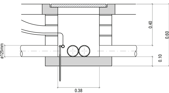
DETALLE DE ARQUETA ALUMBRADO DE 40x40 1/15 (cotas en metros)
