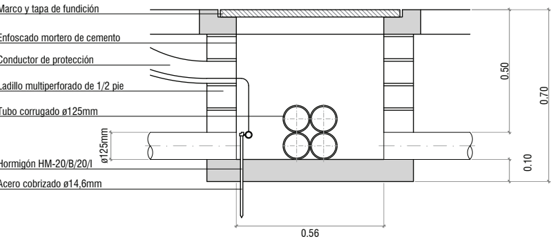
DETALLE DE ARQUETA ALUMBRADO DE 60x60cm 1/15 (cotas en metros)
