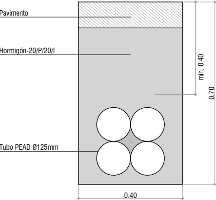
CANALIZACION DE 4 BAJO CALZADA 1/10 (cotas en metros)
